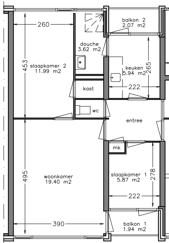
woonlaag 1
