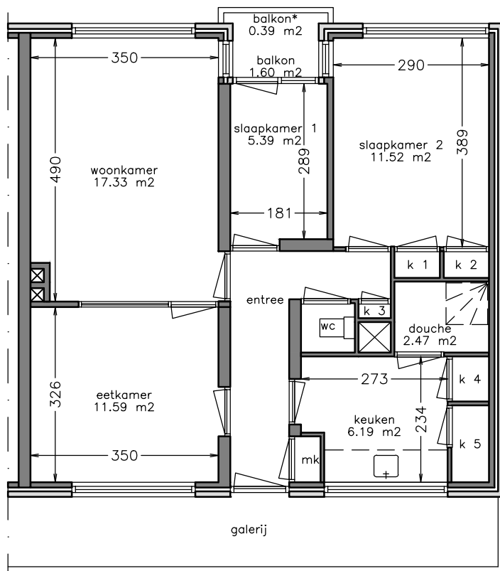
woonlaag 1
