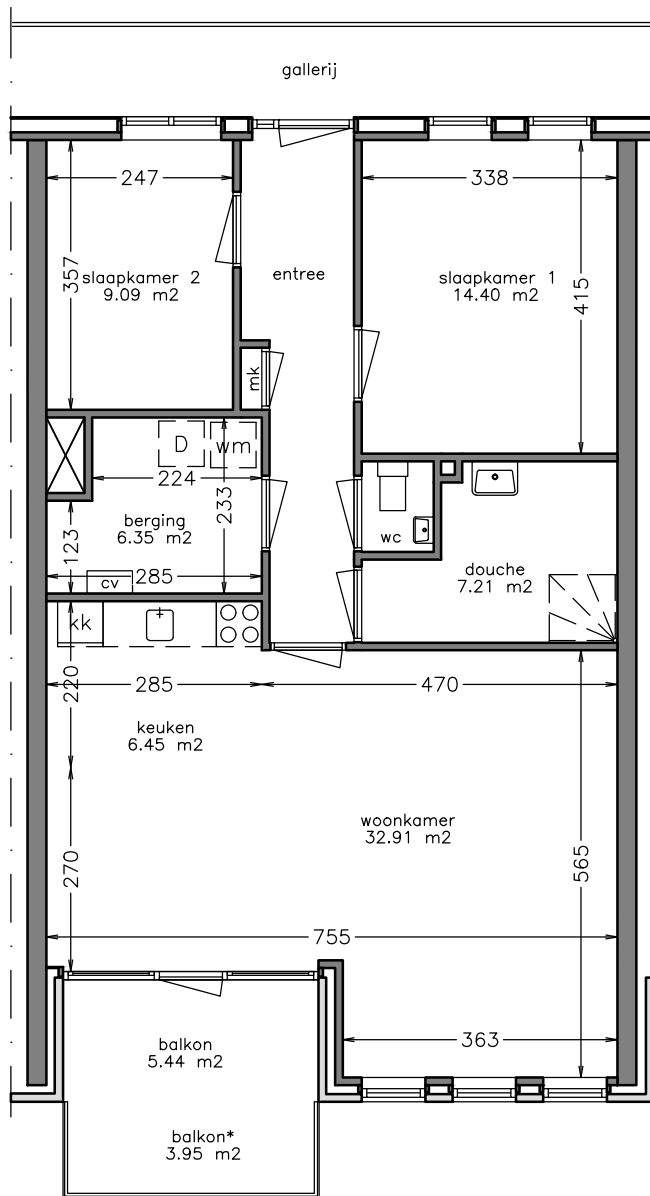
woonlaag 1
