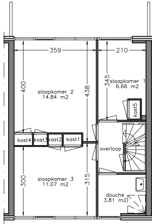
1e verdieping
