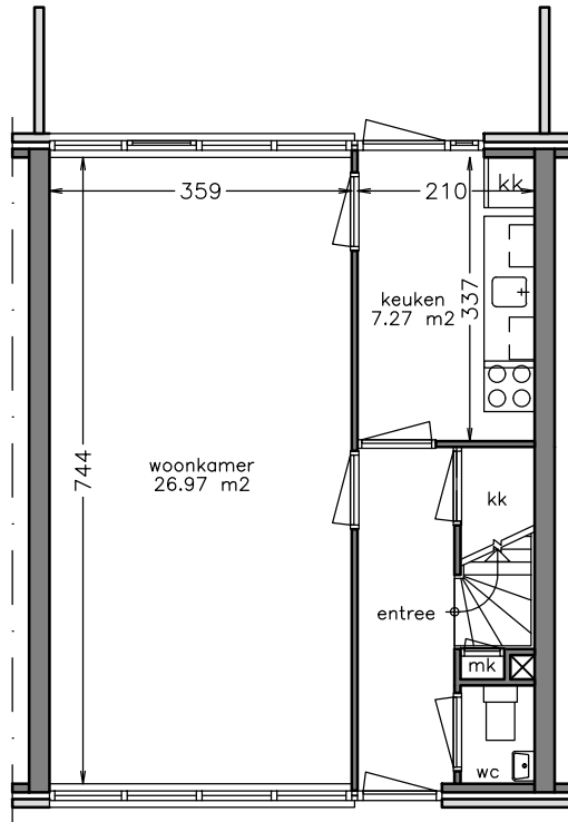
begane grond
