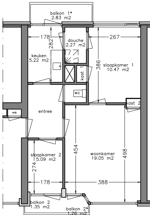
woonlaag 1t/m 3
