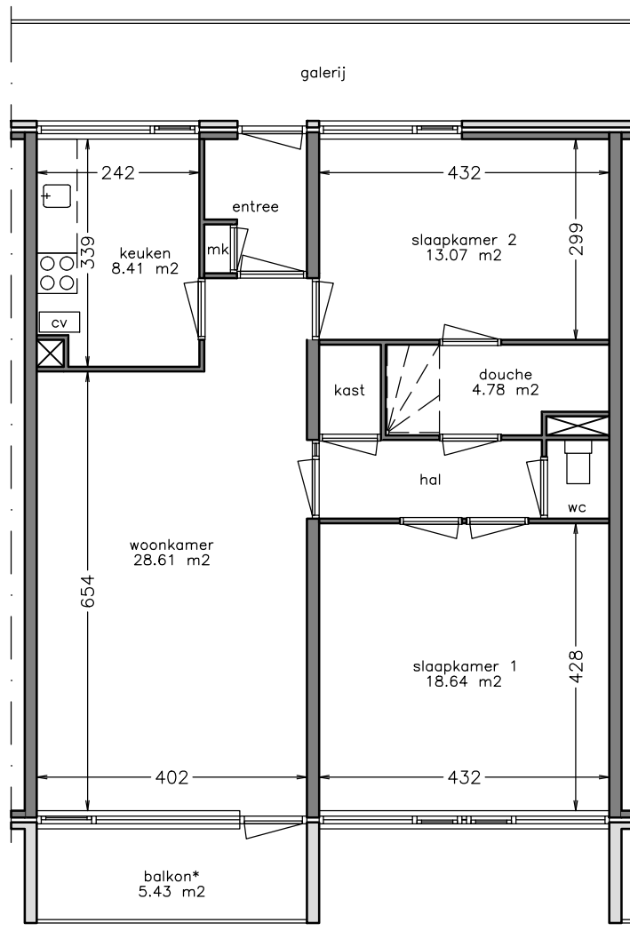
woonlaag 1
