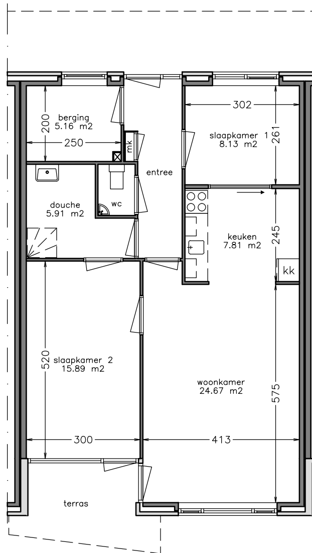
woonlaag 1
