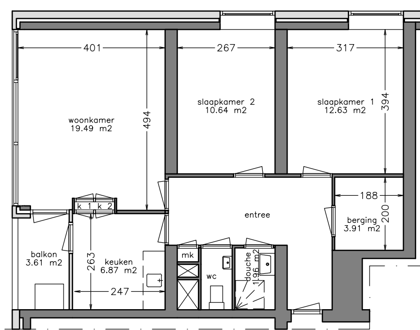
woonlaag 1
