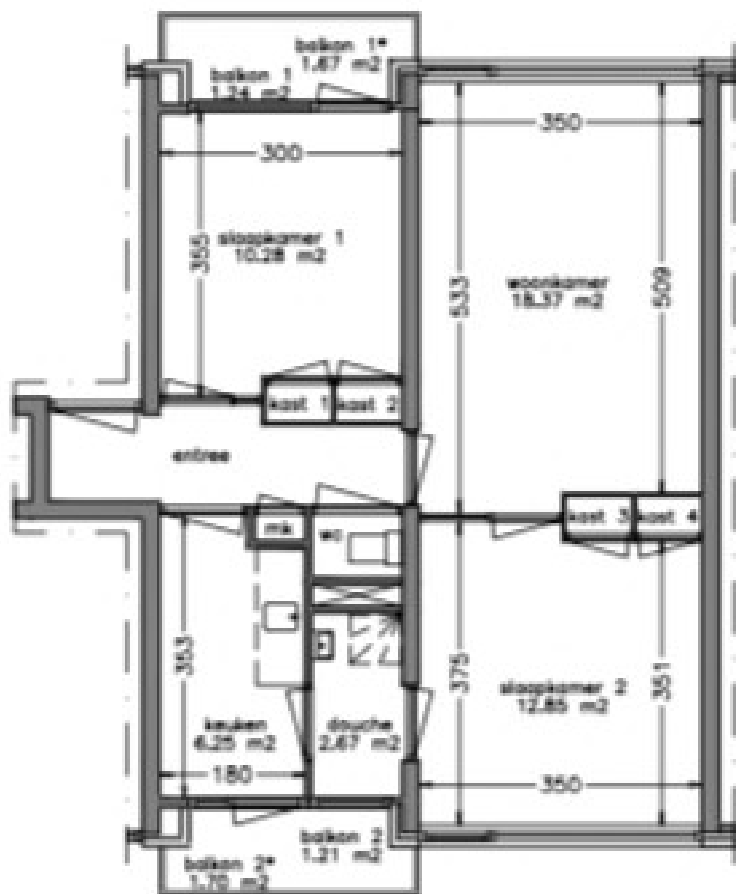
woonlaag 1
