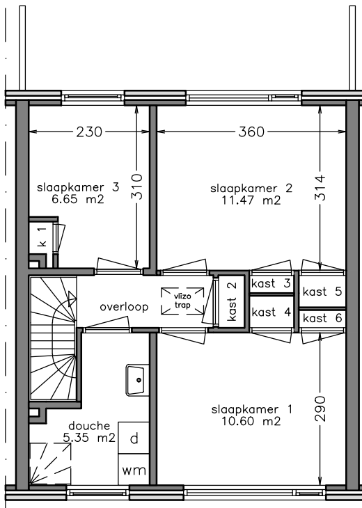
1e verdieping
