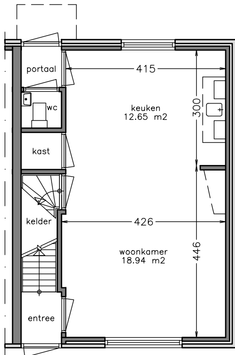
begane grond
