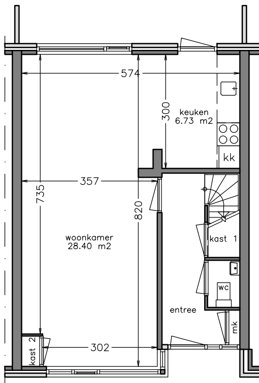
begane grond
