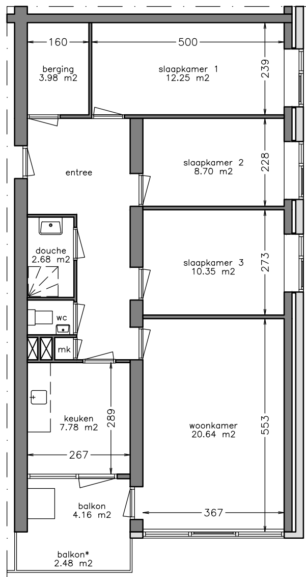
woonlaag 1
