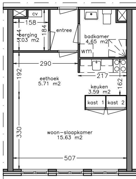
woonlaag 1
