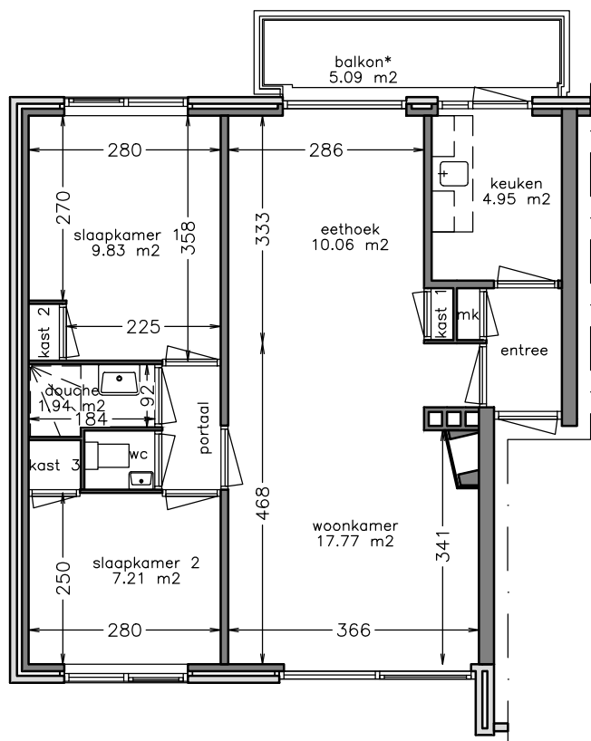
woonlaag 1
