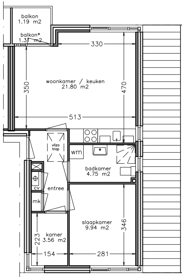
1e verdieping
