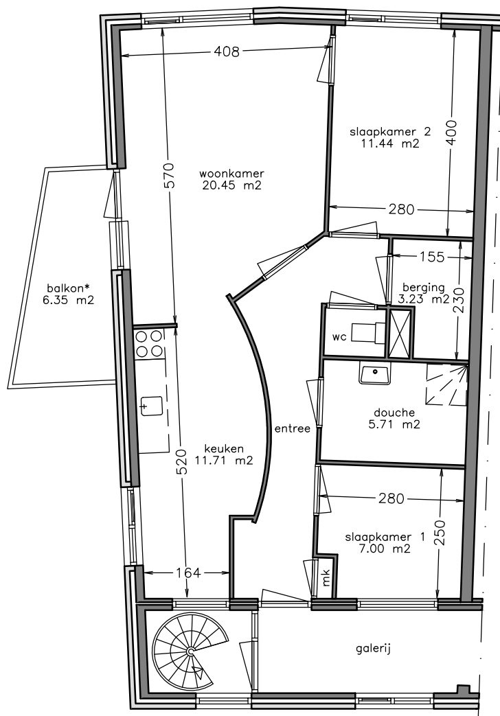
woonlaag 1
