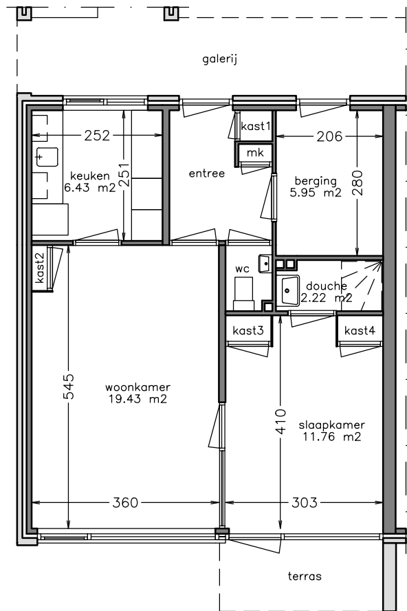
begane grond
