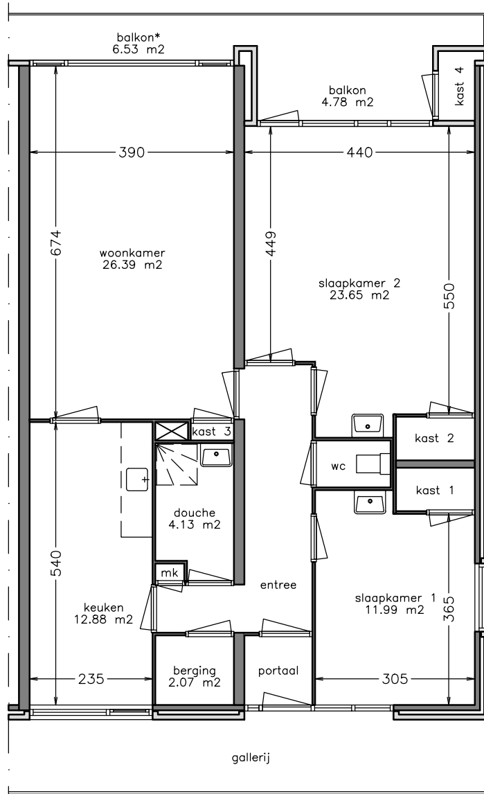
woonlaag 1
