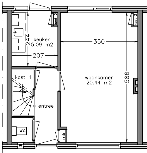
begane grond
