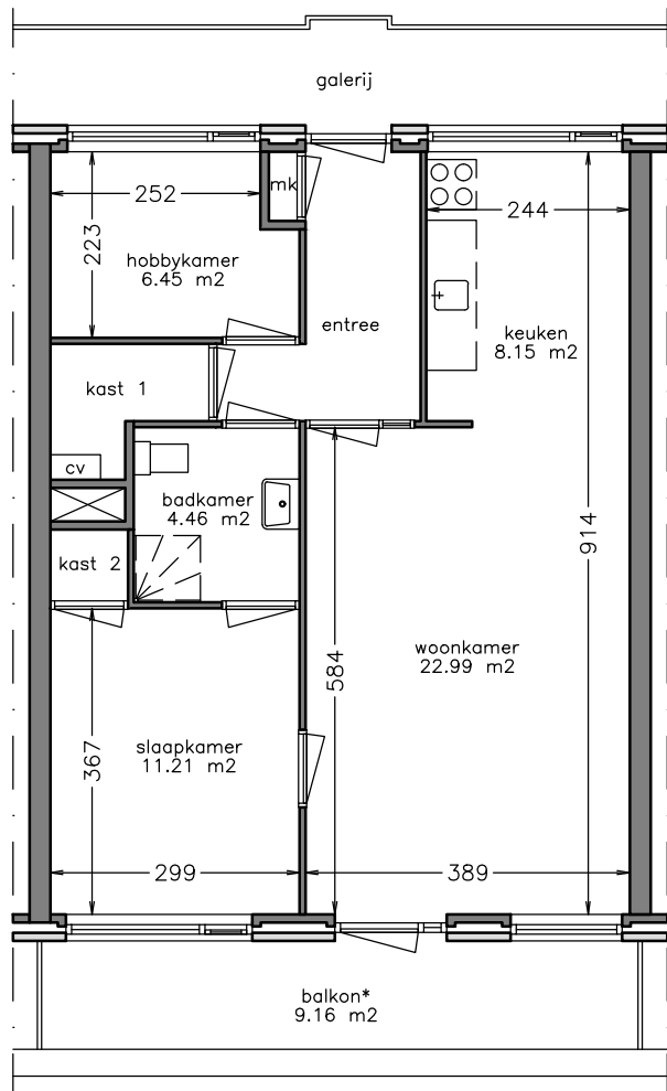
woonlaag 1
