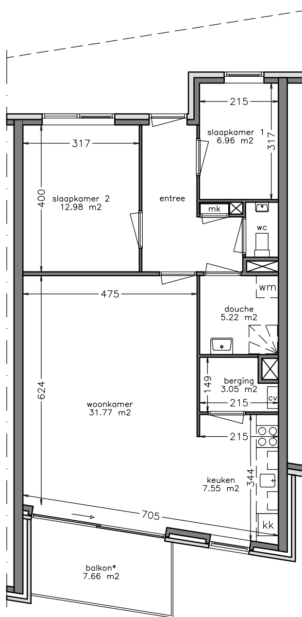
woonlaag 1
