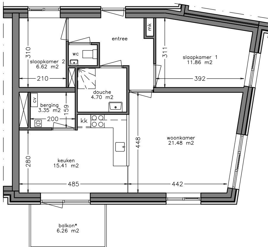
woonlaag 1
