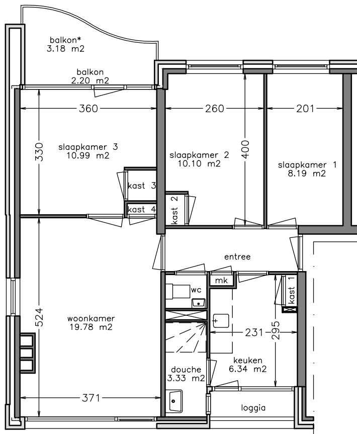
woonlaag 1
